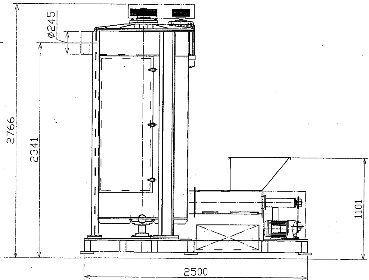
脱水乾燥機
